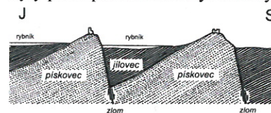
Příčný řez geologickým podložím Holanských rybníků (schéma podle Bruno Müllera).
